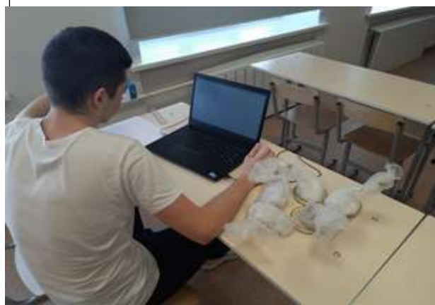
Рис.22- Альбедо снега
